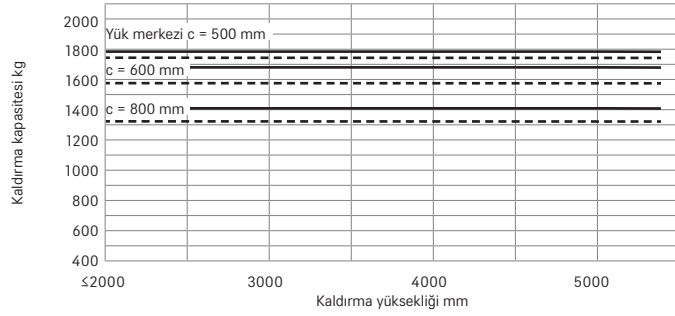
RX 20-18PL Dupleks/HiLo asansör tek SE teker
