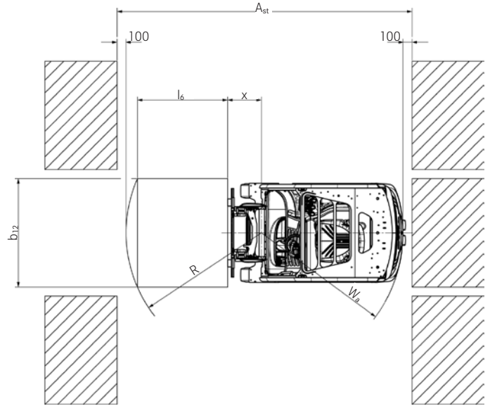
3-teker üstten görünüş
