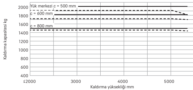
RX 20-20L/RX 20-20PL Dupleks/HiLo asansör tek SE teker
