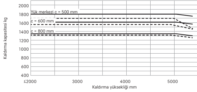
RX 20-18L Dupleks/HiLo asansör tek SE teker
