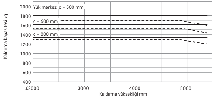
RX 20-20P Dupleks/HiLo asansör tek SE teker
