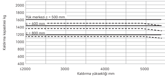
RX 20-16/RX 20-16P Dupleks/HiLo asansör tek SE teker
