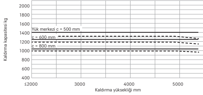
RX 20-16C Dupleks/HiLo asansör tek SE teker
