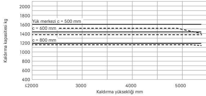
RX 20-16L/RX 20-16PL Dupleks/HiLo asansör tek SE teker
